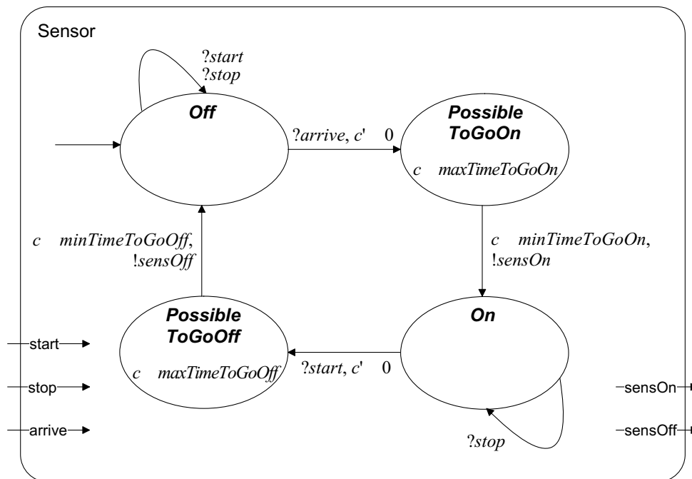
Abbildung 6.12: Sensor-Modul.
